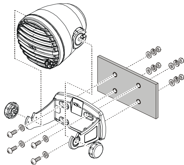
Figure 2 (Wall Mount)
